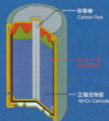
アルカリ乾電池の断面図 Cross-Sectional View of Alkaline Dry Battery
