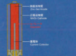
リチウム電池 (コイン型)の断面図 Cross-Sectional View of Lithium Battery
